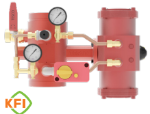
10. 준비작동식 밸브 - 개방형
