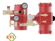
12. 준비작동식 밸브 - 개폐형
